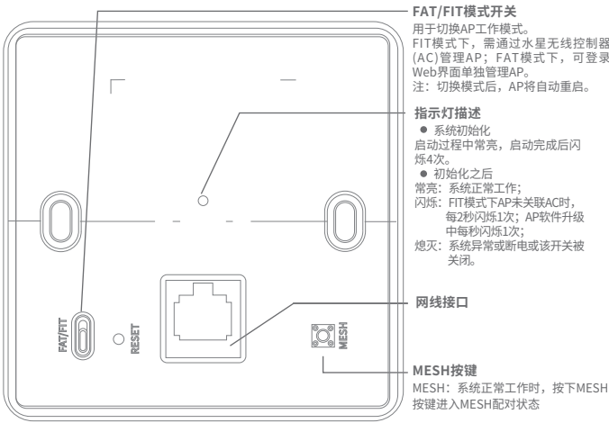
正面示意图
